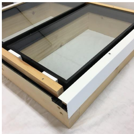
Sidevandnæsen monteres. Skru den evt. for at holde den på plads. Udskæring i sidevandnæsen i forkant
