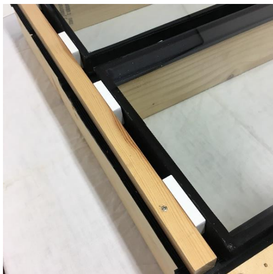
Placering af glasklodse
