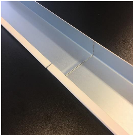
Samling af 2 vandnæser i længderetningen
